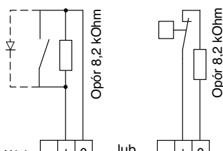
zacisk NO lub dioda LED zabezpieczenia przed zgnieciem
